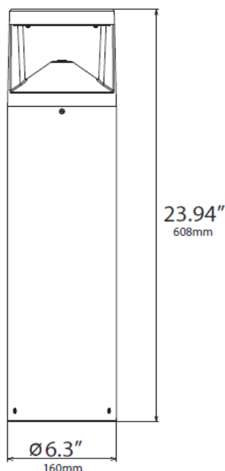
LOC-24BLRD-MW(12/18/24)MCCT(30/40/50)
