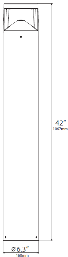
LOC-42BLRD-MW(12/18/24)MCCT(30/40/50)
