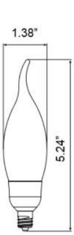
BA11 E12 base
