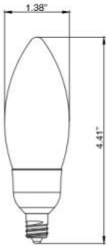
B11 E12 base
