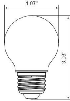
G16.5 E26 base
