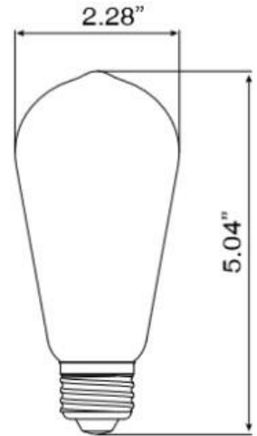
ST19 E26 base
