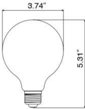
G30 E26 base
